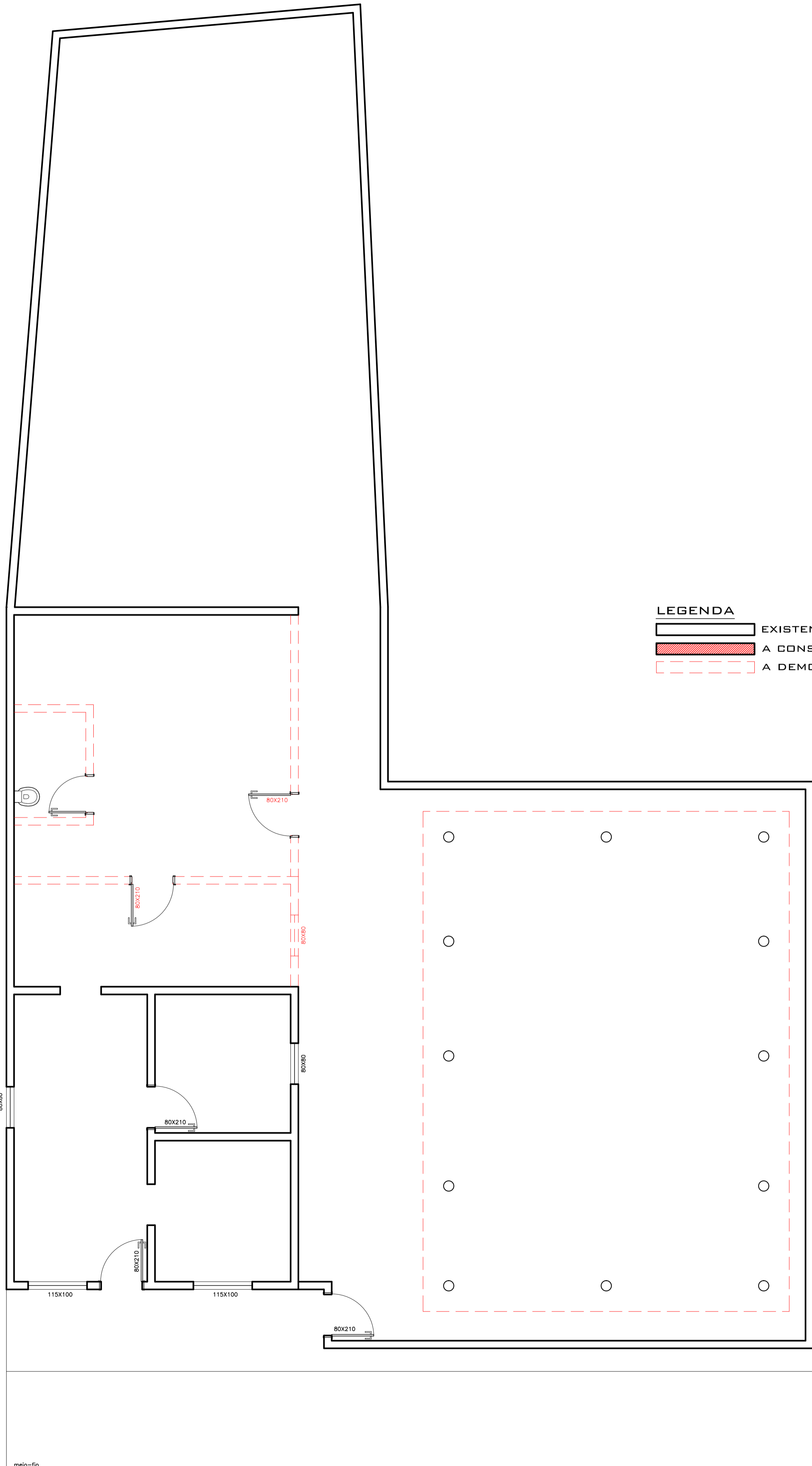
PLANTA Esc. 1:50
