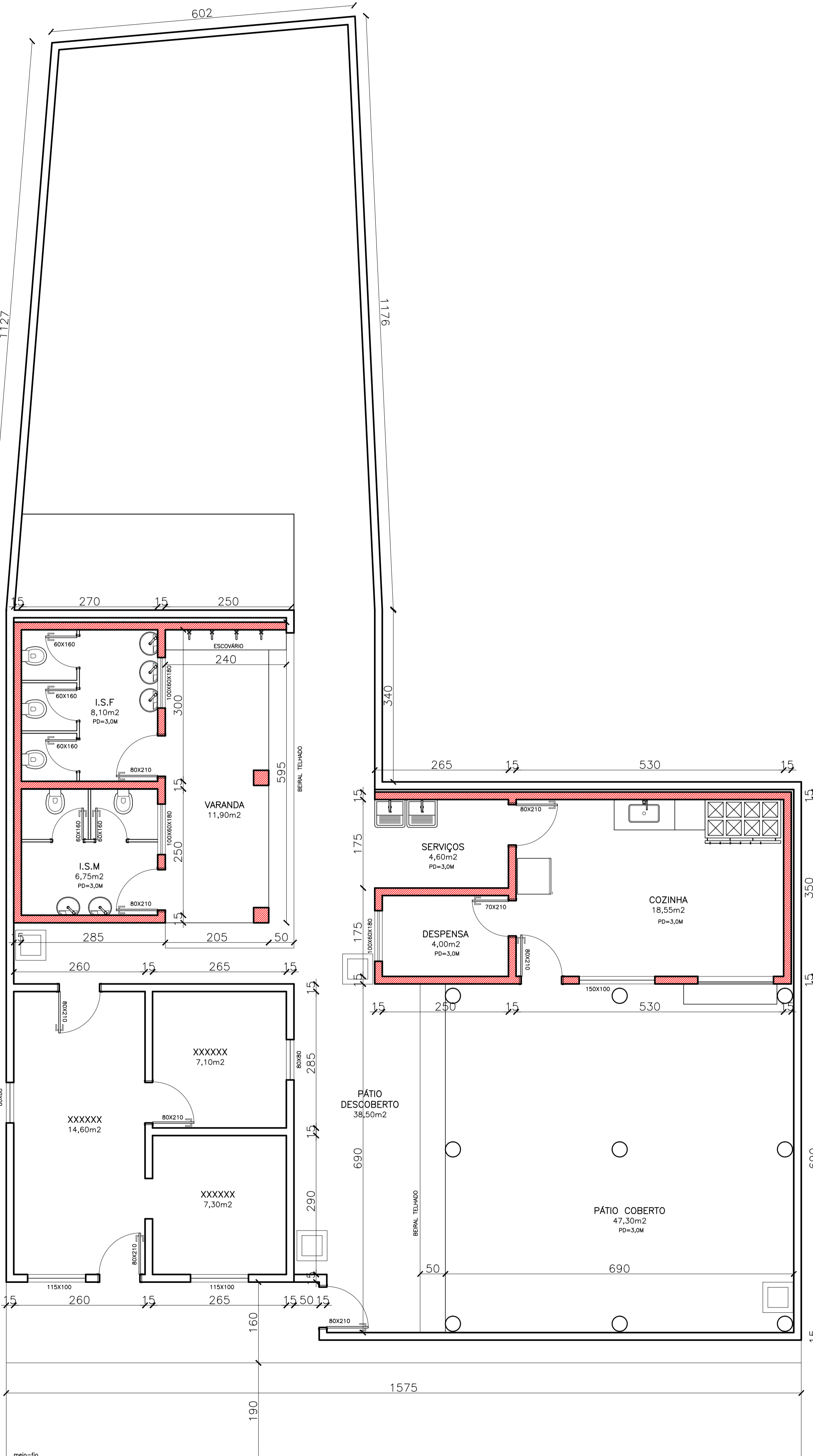
PLANTA Esc. 1:50
