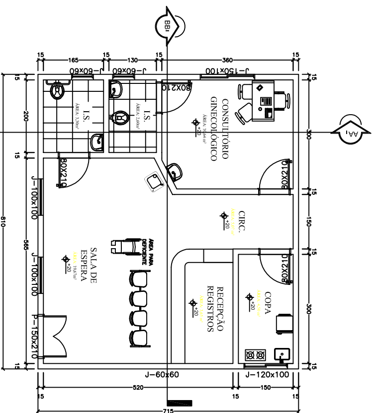
PLANTA-BAIXA Esc.: 1/50
