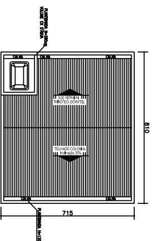
PLANTA DE COBERTURA Esc.: 1/100
